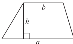
Трапеция
